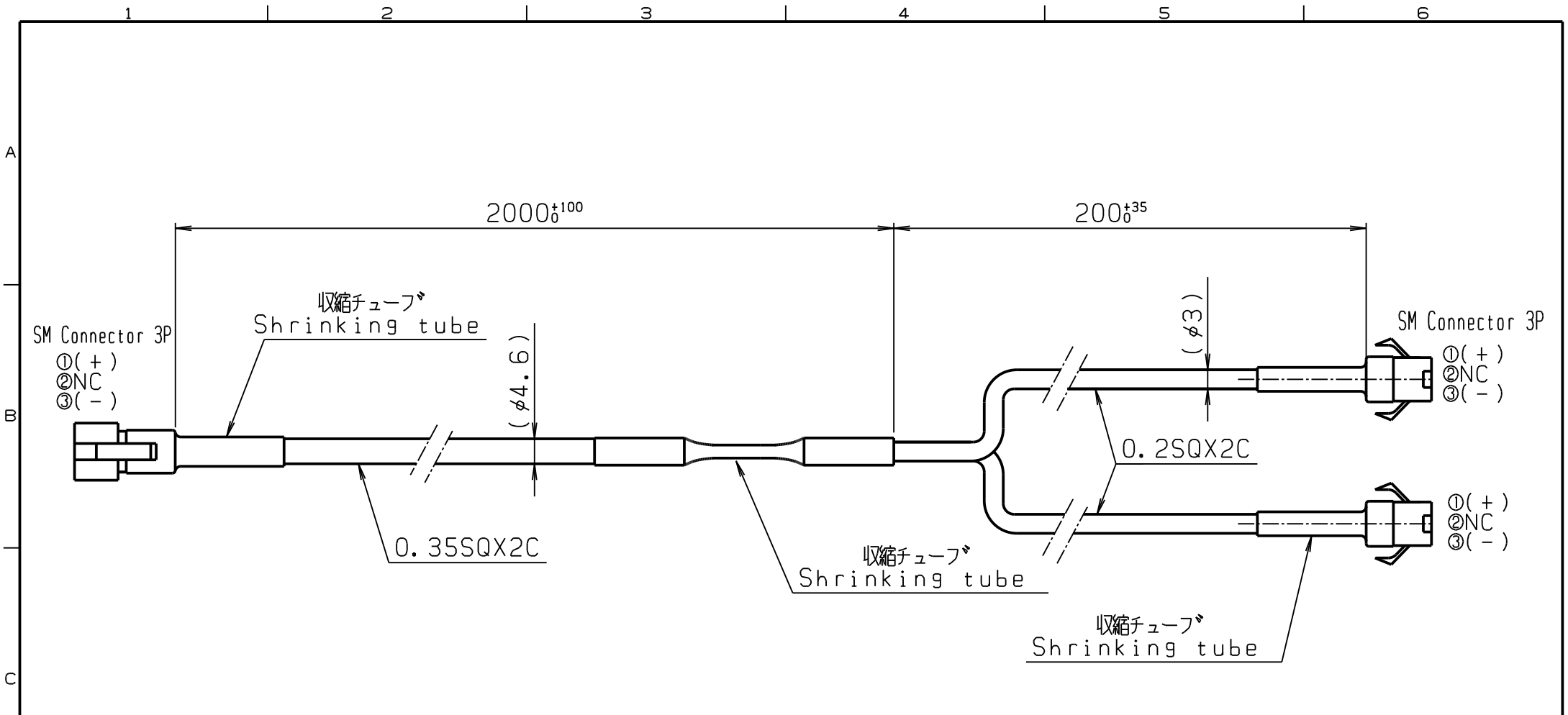
接合部結線 _Connection diagram
